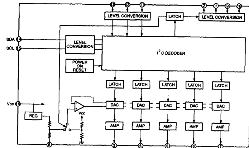
AV BOARD: IC1901 CXA1315M
